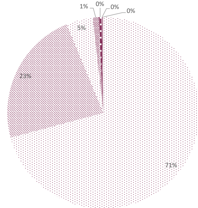
Emisións de CO2 por sectores. Ano 2011. Fonte: PACES Carballo.
